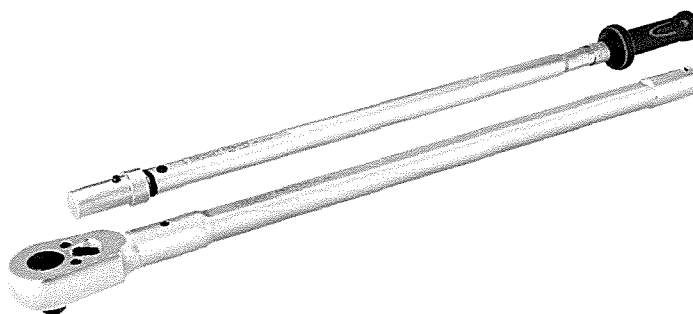
Рисунок 15 – Общий вид ключей моментных предельных HAZET мод. 6150-1СТ, 6160-1СТ
