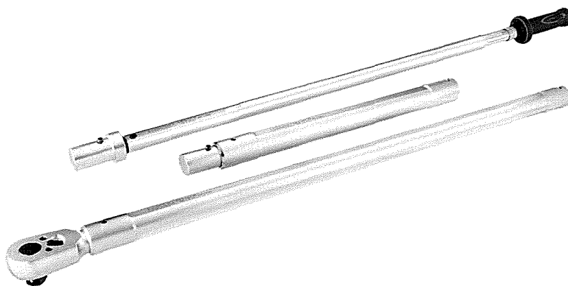
Рисунок 14 – Общий вид ключей моментных предельных HAZET мод. 6170-1СТ
